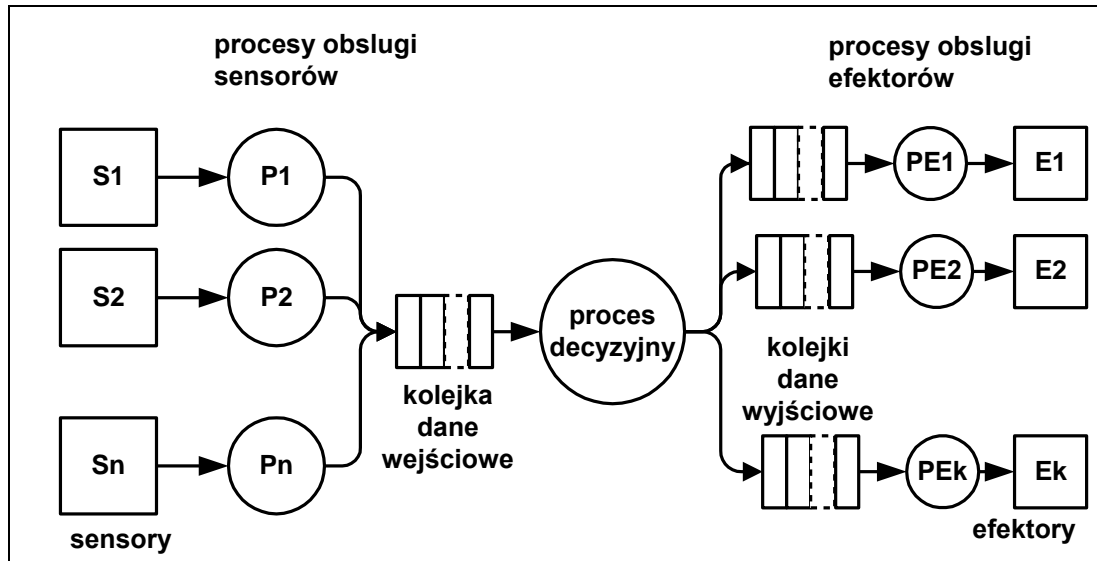
Rys. 1-4 Zastosowanie kolejek komunikatów w robotyce
