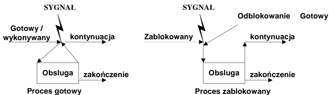
Rysunek 1-1 Obsługa sygnału dla przypadków gdy proces jest gotowy i zablokowany
