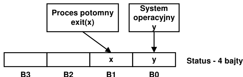
Rys. 2-8 Przekazywanie statusu do procesu potomnego
