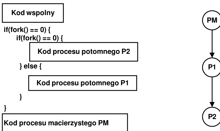
Rys. 2-4 Schemat użycia funkcji fork do utworzenia dwu procesów potomnych P1 i P2. Proces P2 jest procesem potomnym procesu P1.
