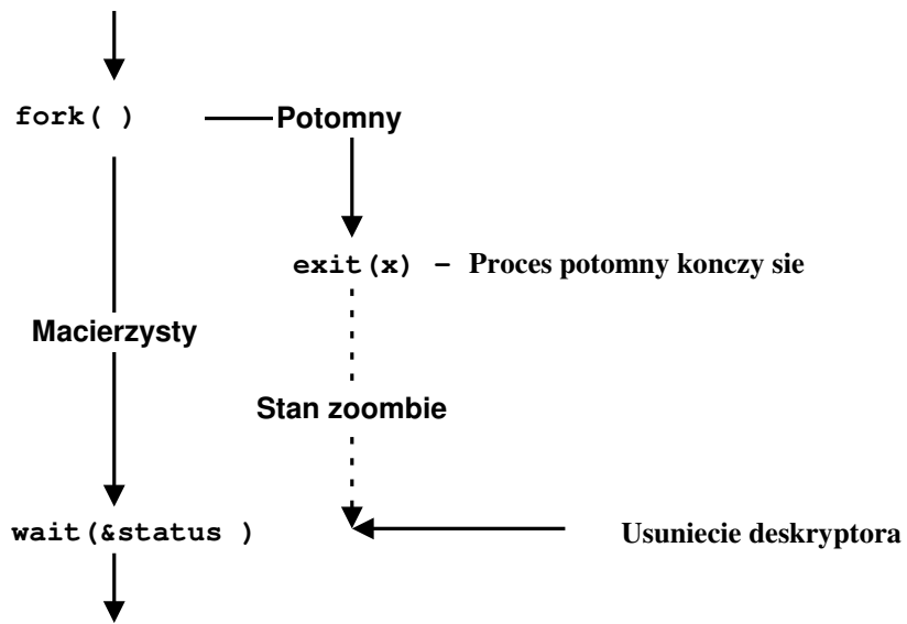
Rys. 2-7 Proces potomny kończy się wcześniej niż proces macierzysty
