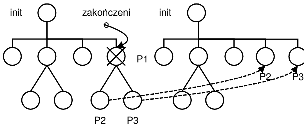
Rys. 2-5 Procesy P2 i P3 adoptowane przez proces init
