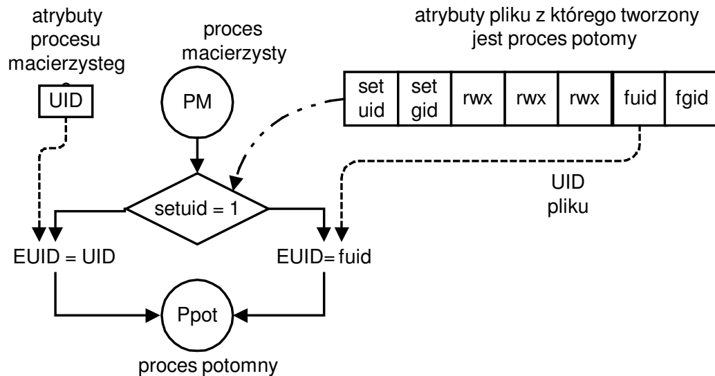
Rys. 2-10 Ustalanie EUID procesu potomnego
