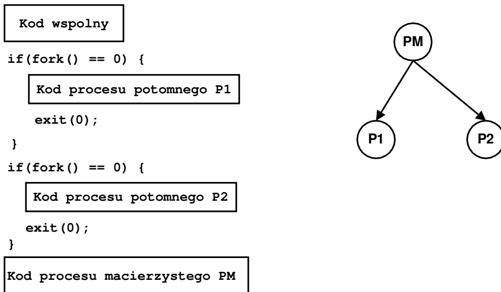
Rys. 2-3 Schemat użycia funkcji fork do utworzenia dwu procesów potomnych P1 i P2. Procesy są utworzone na jednakowym poziomie hierarchii.
