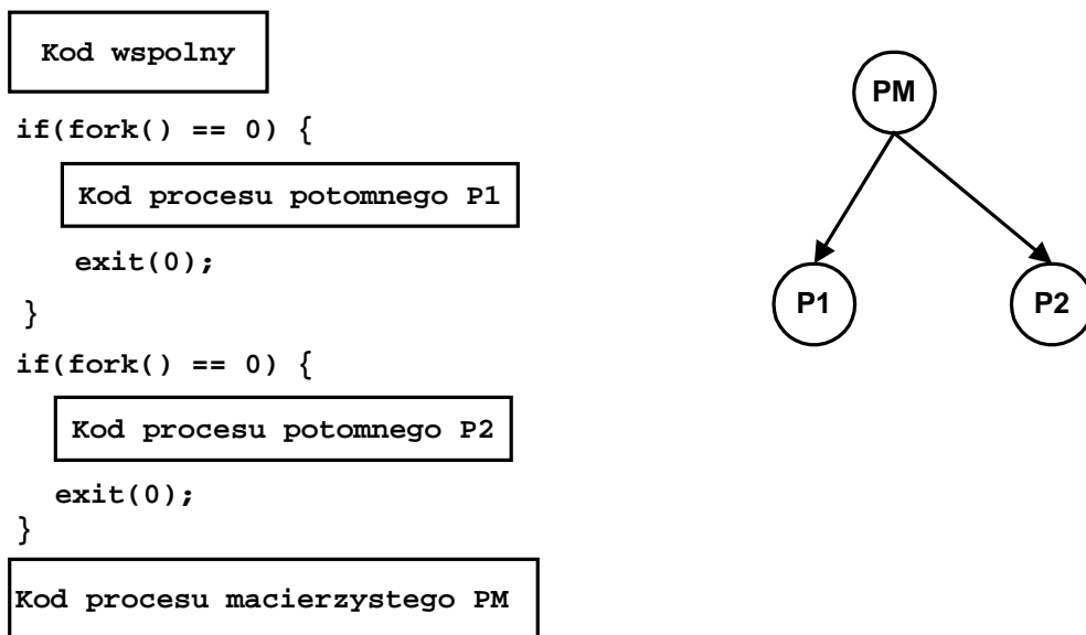
Rys. 2-4 Schemat użycia funkcji fork do utworzenia dwu procesów potomnych P1 i P2. Procesy są usytuowane na jednakowym poziomie hierarchii.
