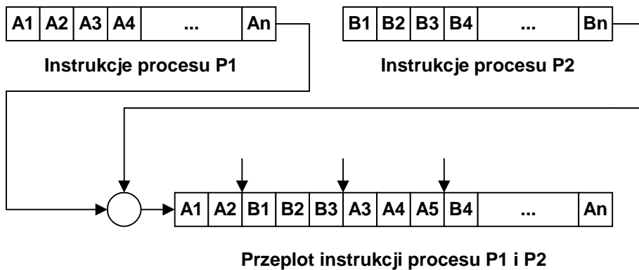
Rys. 9-2 Instrukcje procesów P1 i P2 wykonywane w trybie przeplotu
